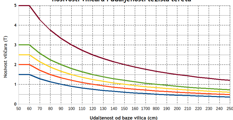
Nosivost produžnih vilica u ovisnosti o nosivosti viličara i udaljenosti težišta tereta
