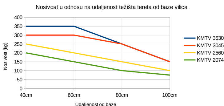
KMTV dijagram nosivosti
